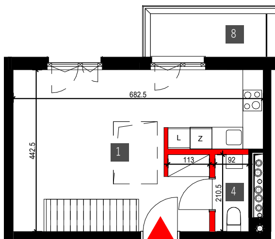
kondygnacja +3
