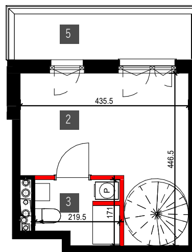
kondygnacja +2
